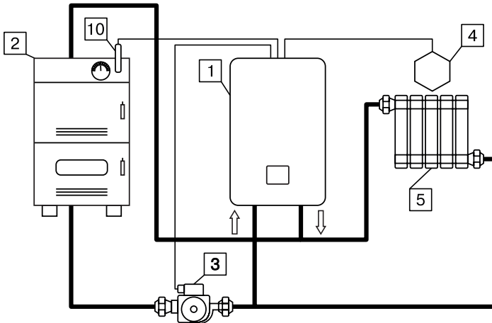
Рис.7 Упрощенная схема подключения миникотельной в режиме вспомогательной.
